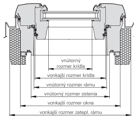
rez B-B
