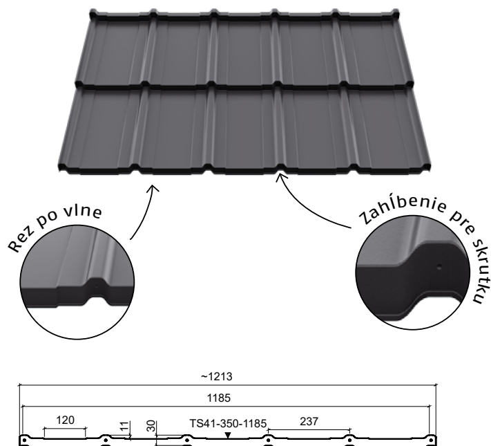
Pohľad čelný
