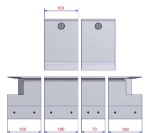
Fensterbankeinsatz Variabel
