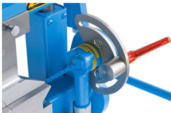
Biegewinkelbegrenzungsanschlag (Serienausstattung)
