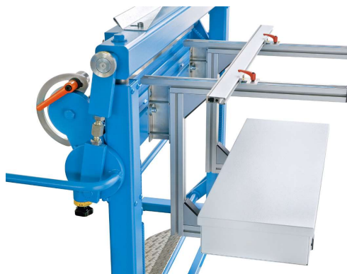
manueller Tiefenanschlag mit Alu-T-Nut
