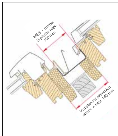
Rez oknom R4/R7
