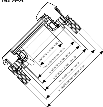
rez A-A
