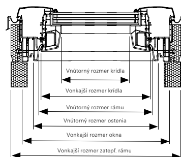
rez B-B
