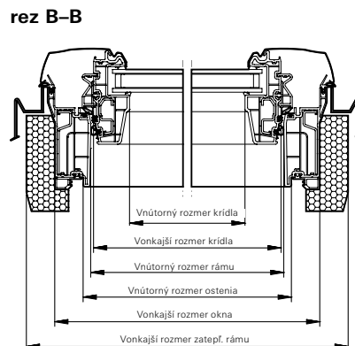
rez B-B
