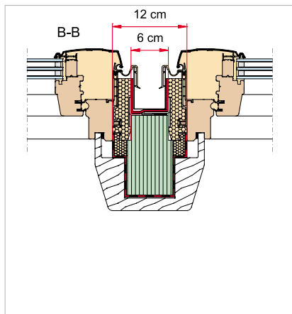
Kombinácia pomocnej krokvy EKS s obložením z masívneho dreva v bielej farbe pre iný systém ostenie než Roto ZIN
