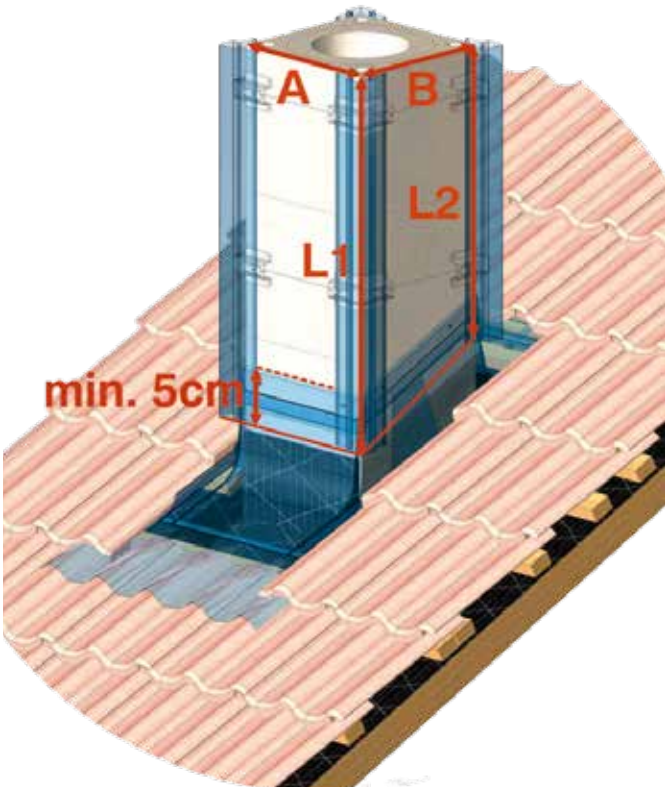
Samo-upínací systém
