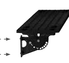
Držiak na snehovú mrežu, hliník Funkcia: 4071/4060
